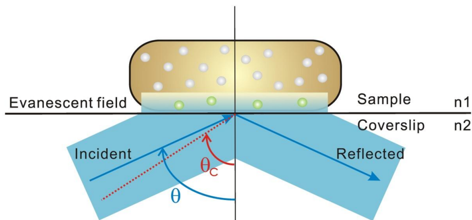
TIRF
